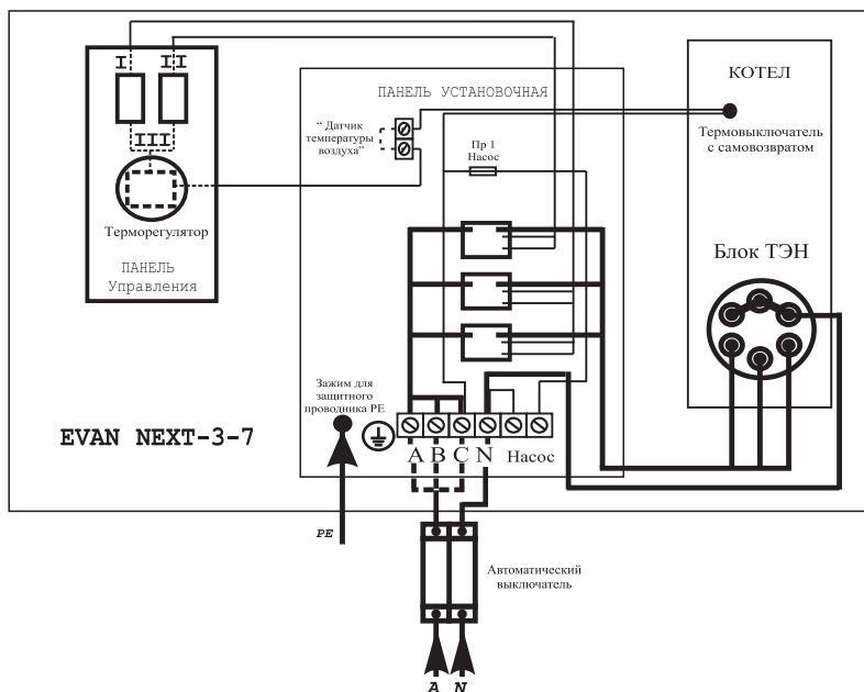
Рисунок 5. Электрическая схема подключения EVAN NEXT-3-7/220
