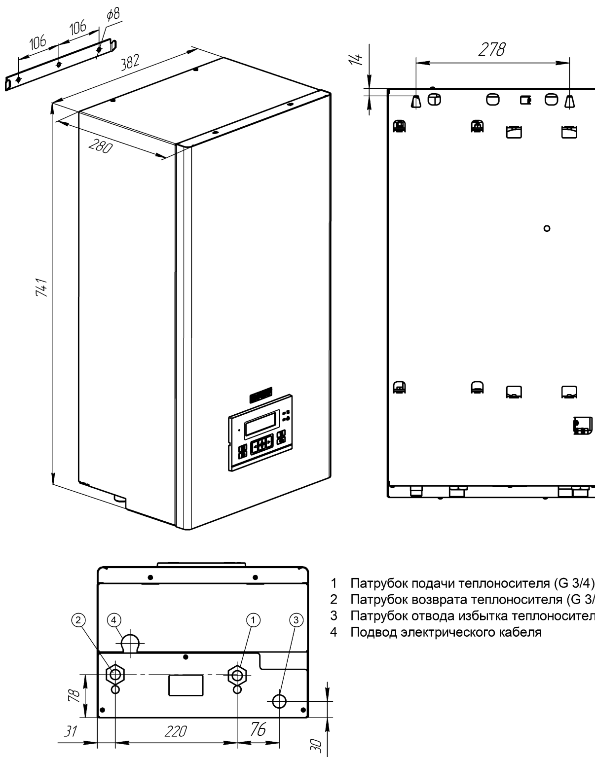
Рисунок 20. Габаритные и присоединительные размеры прибора
