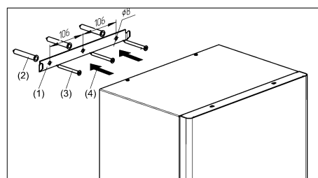
Рисунок 4. Установка прибора на вертикальное основание
