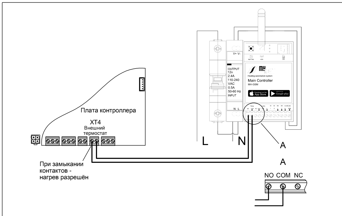
Рисунок 35. Схема подключения контроллера MyHEAT GSM по релейному выходу
