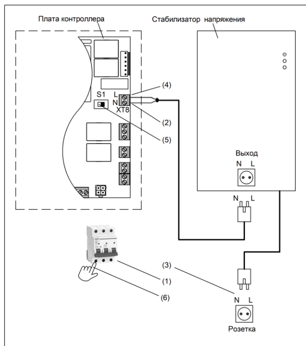
Рисунок 27. Схема подключения стабилизатора напряжения
