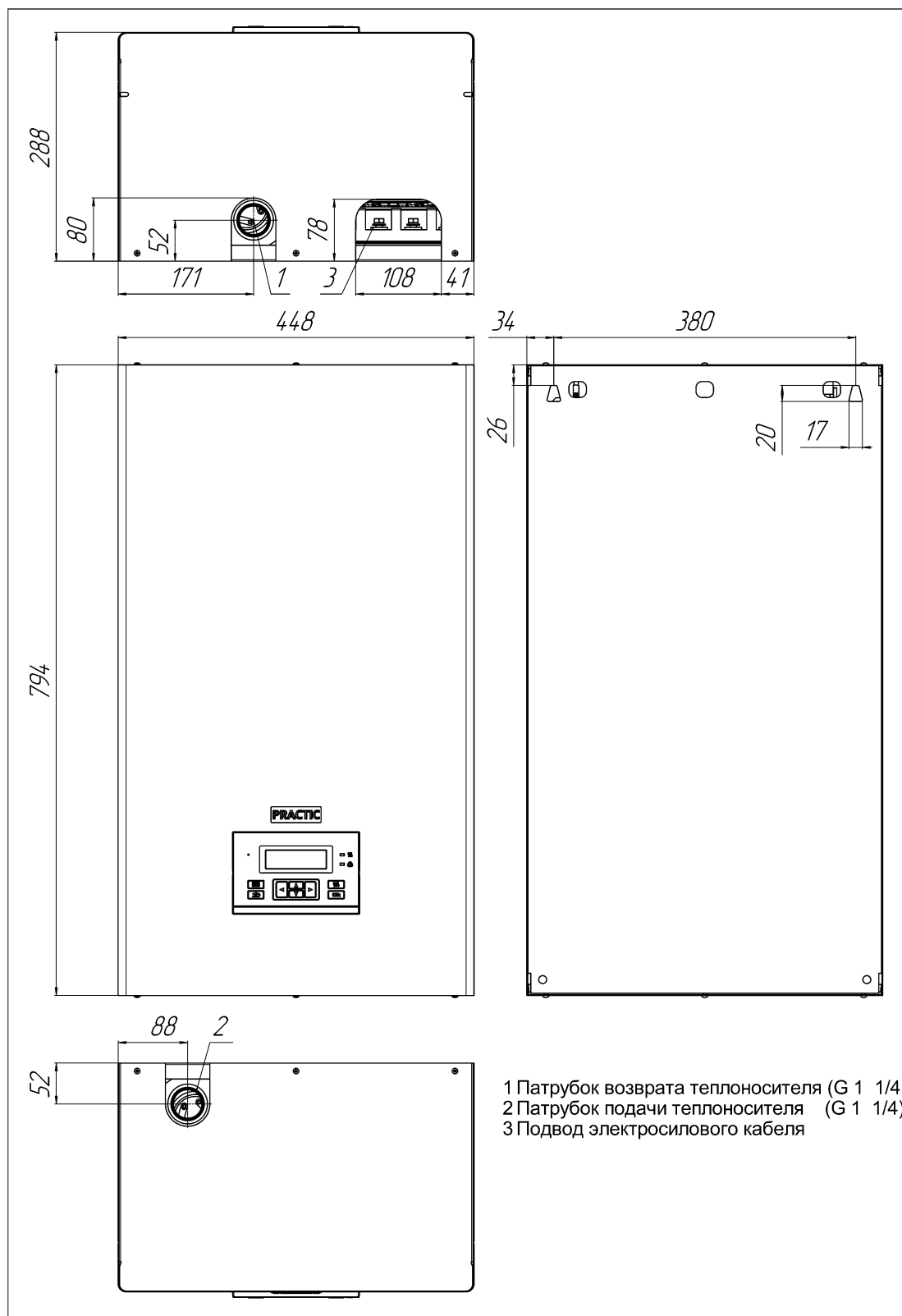
Рисунок 20. Габаритные и присоединительные размеры приборов ЭВАН PRACTIC-36,....., PRACTIC-120
