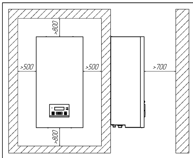
Рисунок 3. Минимальные расстояния
