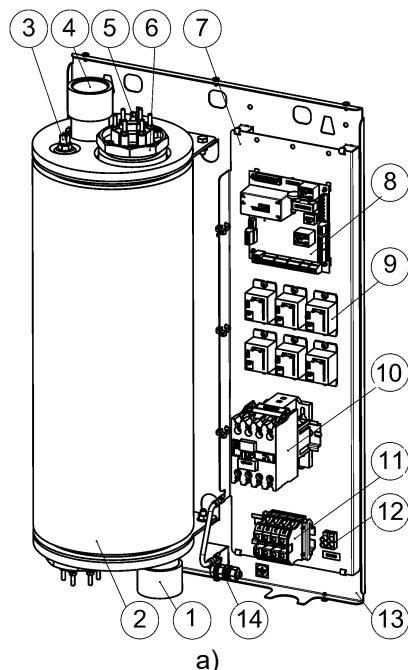
Рисунок 2. Общий вид прибора (кожух, блок управления условно не показаны)
