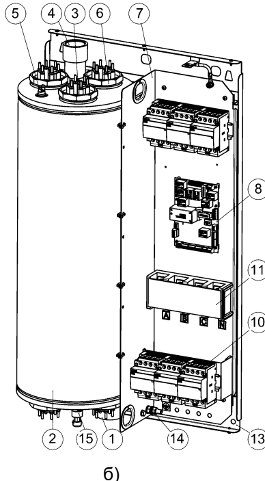
Рисунок 2. Общий вид прибора (кожух, блок управления условно не показаны)
