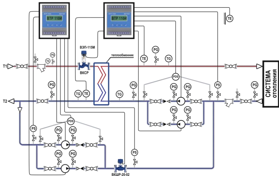
Рисунок Б.2 – Монтажная схема регуляторов ВТР 110И в системе управления независимым контуром отопления (программа 10) и контуром подпитки (программа 40)
