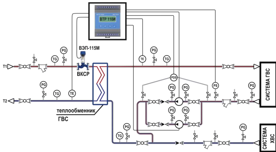
Рисунок Б.3 – Монтажная схема регулятора ВТР 110И (программа 20) в системе управления контуром ГВС
