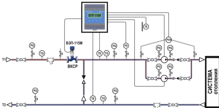
Рисунок Б.1 – Монтажная схема регулятора ВТР 110И (программа 10) в системе управления зависимым контуром отопления
